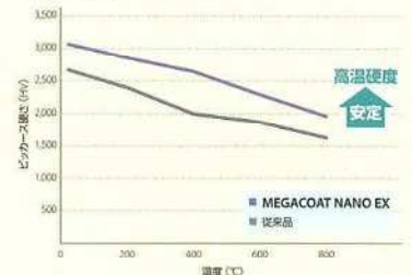
ピッカース硬さの温度推移 (当社比較)
